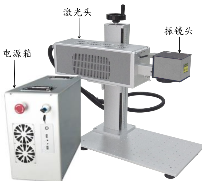
E 系列 CO 2 激光打标机
