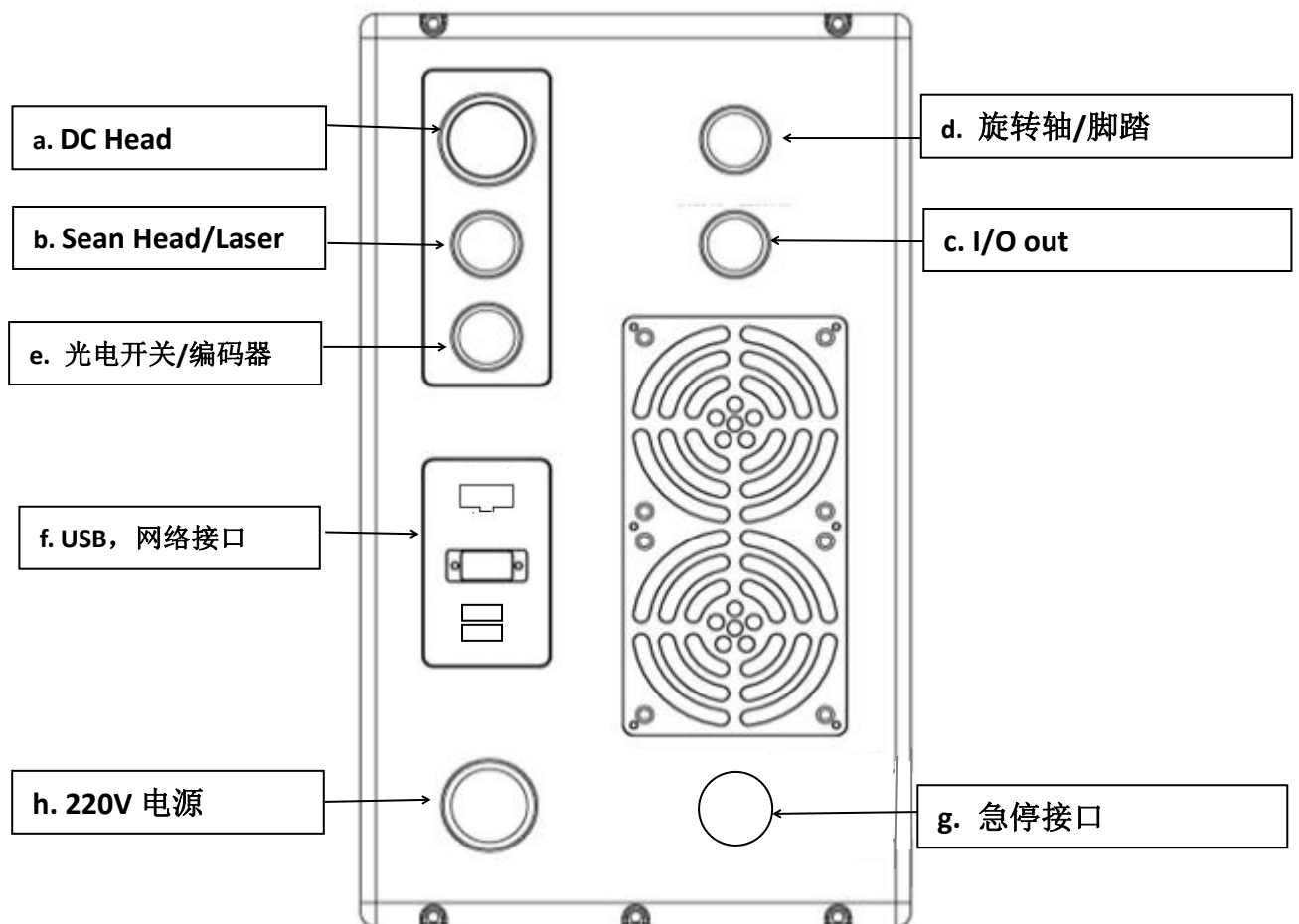
电源箱后面板
