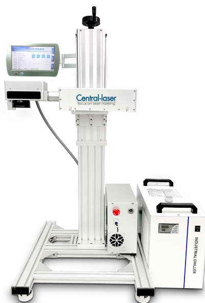
图 1：打标机整体结构
